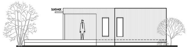
end elevation
